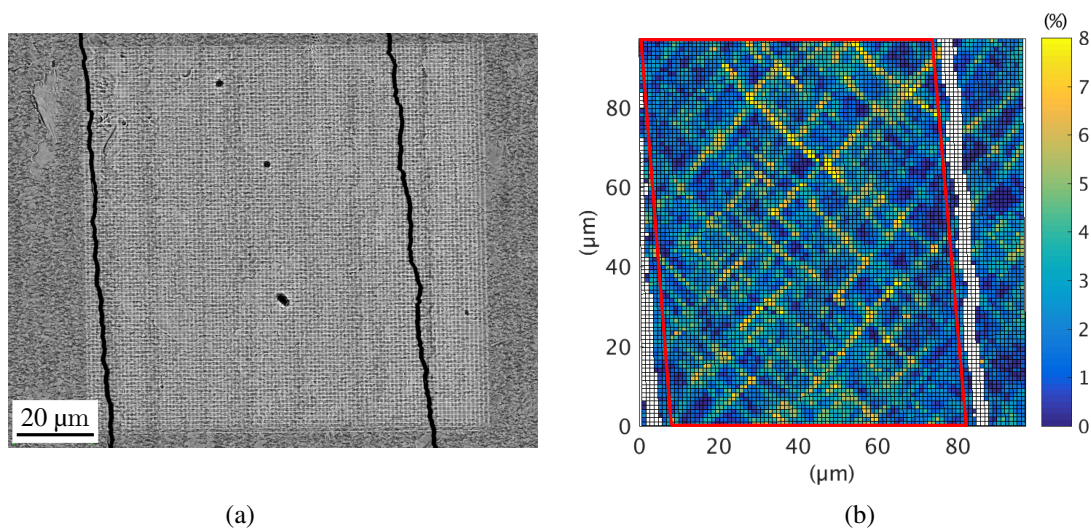
FIGURE 8 – (a) Image de la microgrille traversée par deux fissures transversales. (b) Cartographie de la déformation à la surface du revêtement selon la direction de traction, à la dernière interruption.
