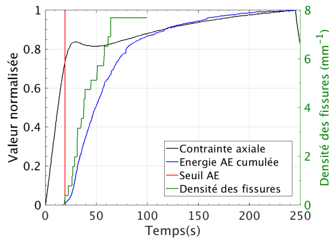
FIGURE 5 – Évolution de l’énergie cumulée normalisée des signaux acoustiques et de la contrainte axiale globale en fonction du temps dans le cas de la traction simple; seuils d’apparition des premières fissures d’après les mesures de AE. Évolution de la densité des fissures dans la zone observée par la caméra en fonction du temps.
