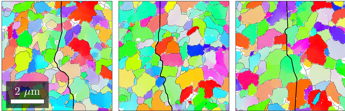
FIGURE 9 – Cartographies EBSD d’orientation cristalline autour de fissures peu ouvertes (illustrées par les lignes noires) (35 nm/pixel).
