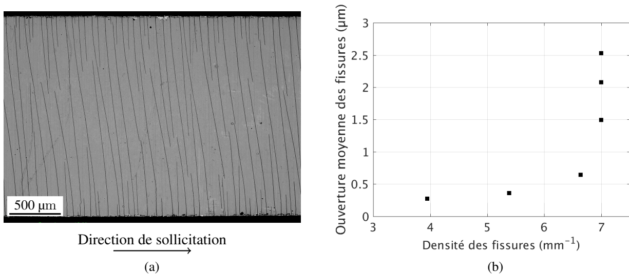
FIGURE 7 – (a) Réseau des fissures à saturation. (b) Evolution de l'ouverture moyenne des fissures en fonction de la densité des fissures selon la direction de traction.
